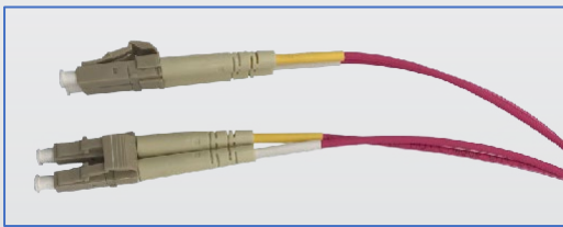
Tapa protectora antipolvo, conector, funda liberadora de tensión, anillo identificativo, tubo termorretráctil, y cable OM4 50/125 LSZH.
