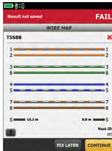
Mapa de cableado: muestra la distancia al error, ruptura o cortocircuito
