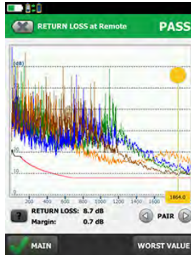
Gráfico de pérdida de retorno
